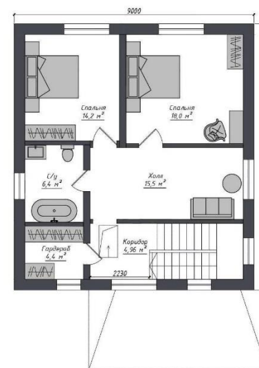
План 2-го этажа
